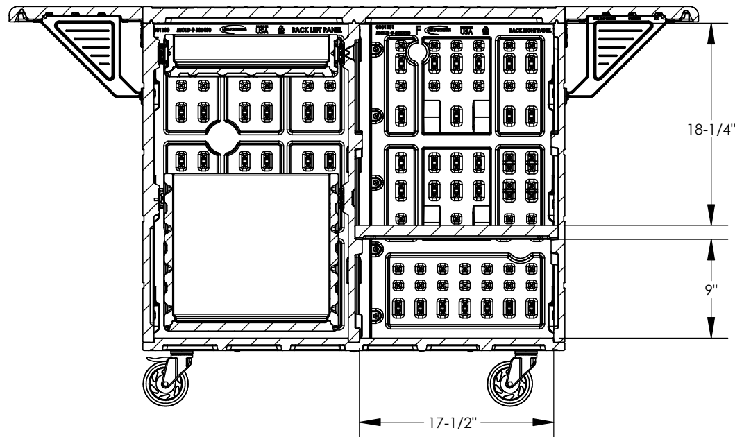
SECTION A-A SCALE 1 : 12
